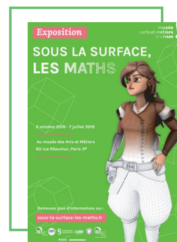
Sous la surface, les maths
